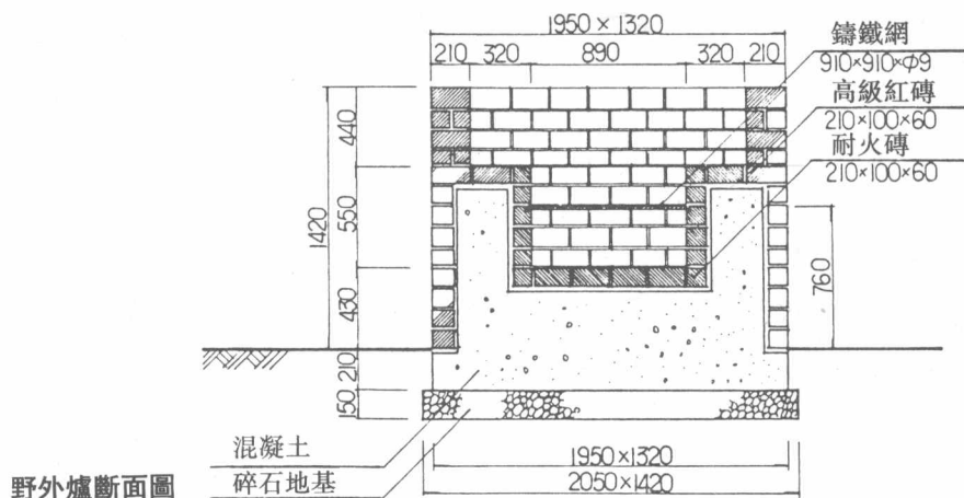
野外爐斷面圖
