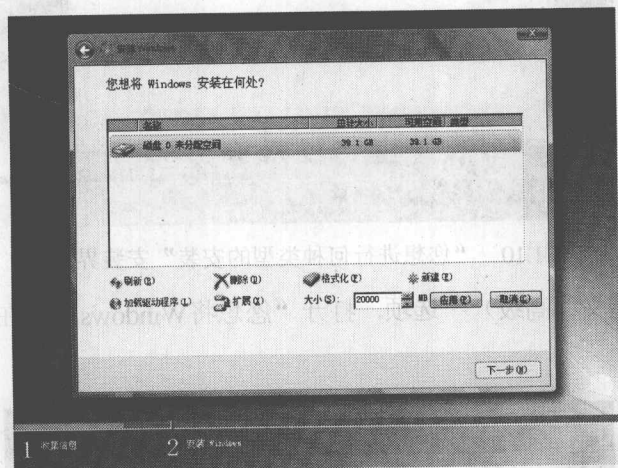
图1.13 输入“20000”
