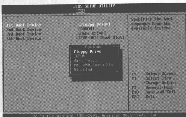
图1.2 “Options”选项框
