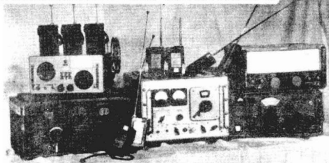
在秘密据点缴获的 部分收发报机
