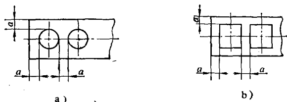
图 11-3 冲裁件内孔之间及孔壁与边缘之间的最小距离
