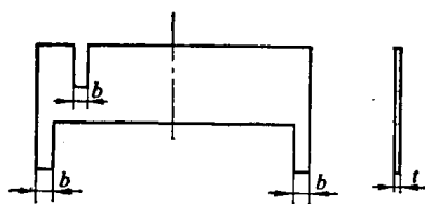
图 11-1 带有悬臂和狭槽的工件
