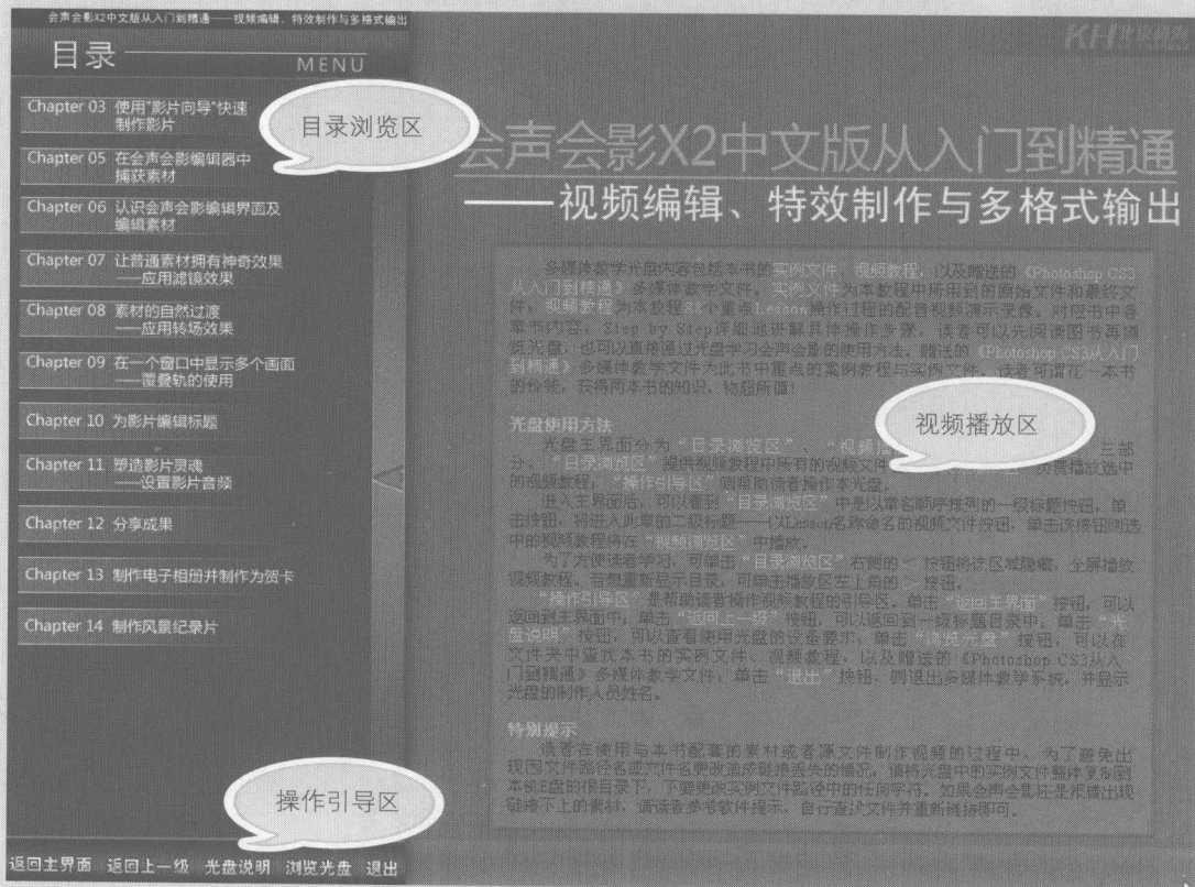
图1 光盘主界面
