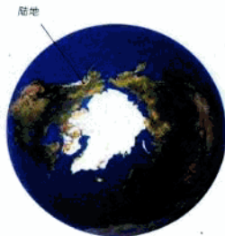
从北极俯视北半球
