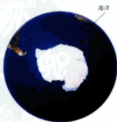
从南极俯视南半球
