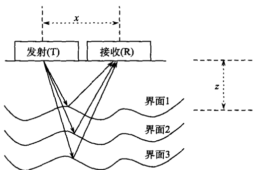
图 1.1 地质雷达野外探测示意图
