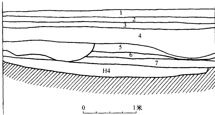
图四 T0302 东壁剖面图
