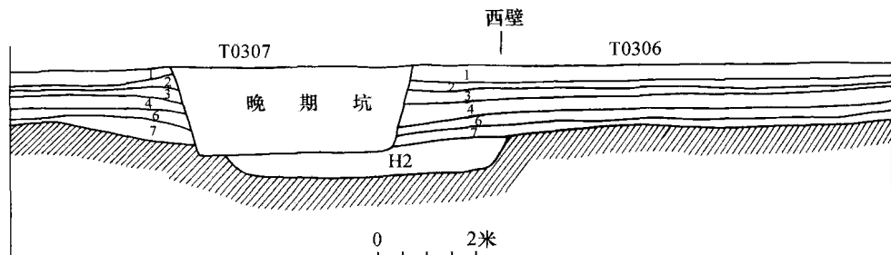
图三 T0307 ~ T0306 西壁剖面图
