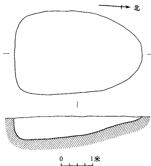
图六 H3 平、剖面图
