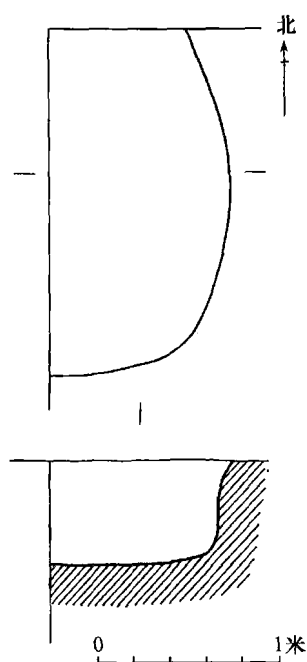
图九 H7 平、剖面图
