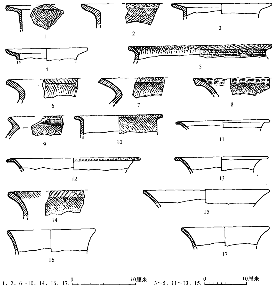
图一二 第7层出土陶器
