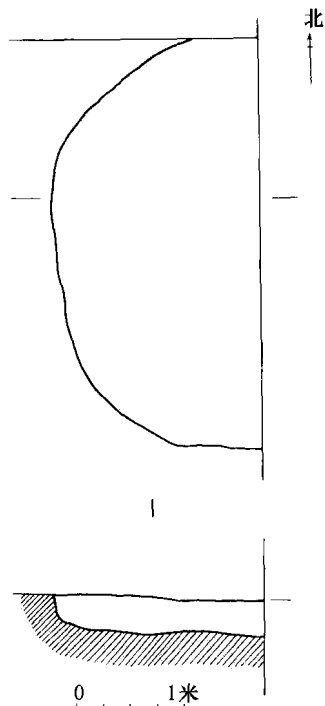
图七 H4 平、剖面图
