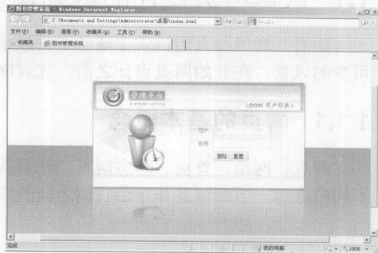
图1-5 动态网页
