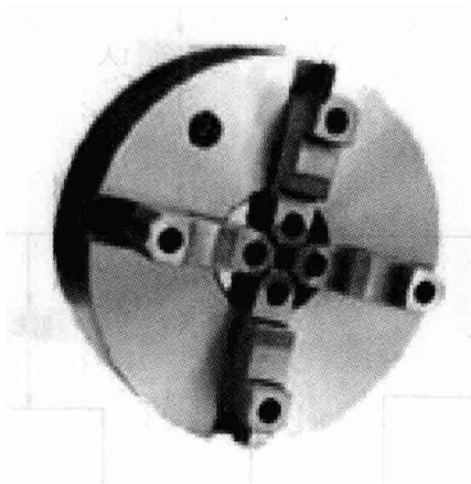
图 2-2 高档卡盘 K88 2500 实物图
