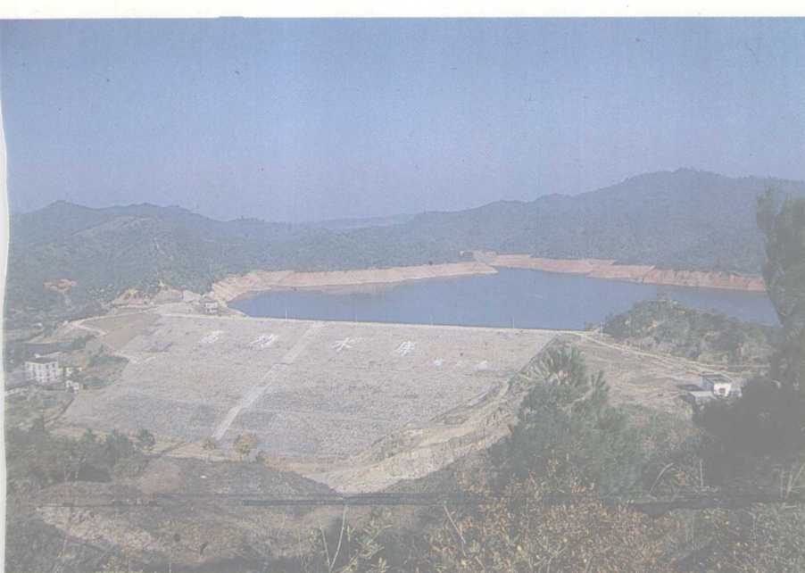
高坊水库——1958 年动工兴建，1960 年开始蓄水，库名 由全国政协副主席 钱正英题写。
