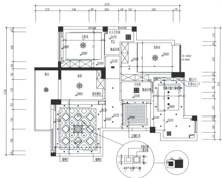
吊顶布置图
