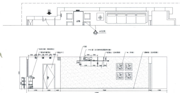
立面图2
