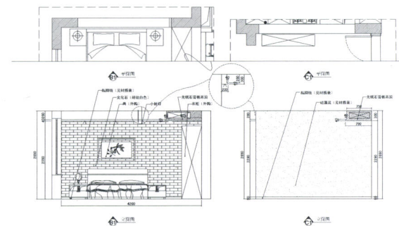
立面图3
