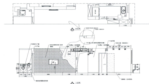
立面图1
