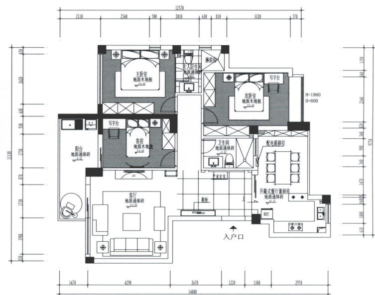
平面图
