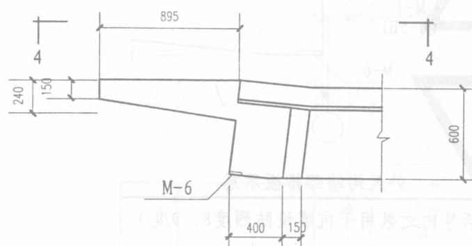
自由落水端节点模板图
