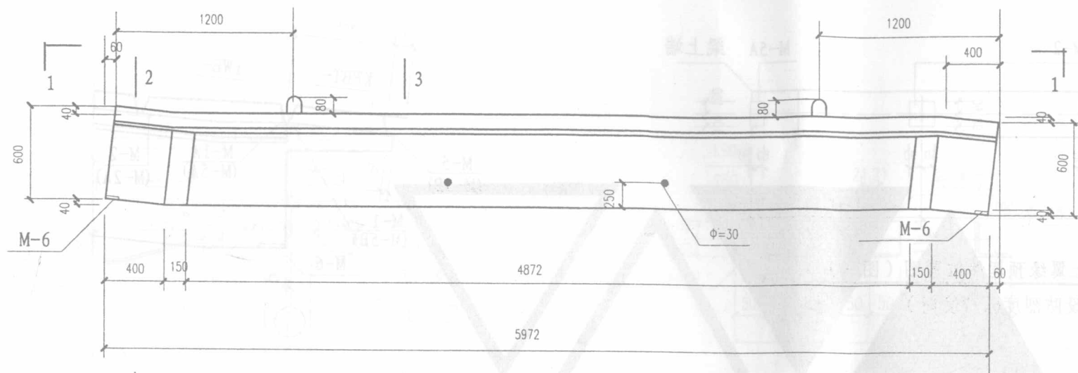
模板图 (无天沟端节点)
