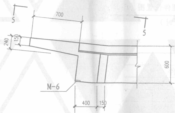
外天沟端节点模板图
