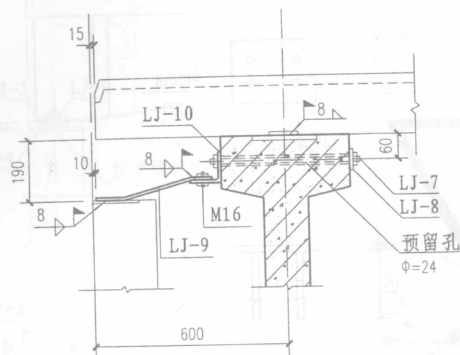
山墙柱与屋面梁连接节点示意
