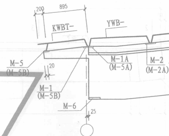
自由落水端部排板示意
