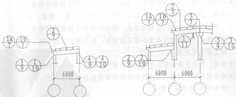
构件布置示意图 (抗震设防烈度为 8、9 度)
