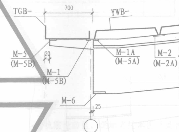
外天沟端部排板示意
