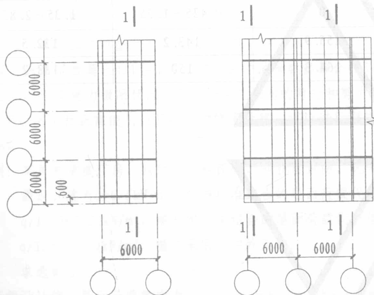
构件平面布置示意图
