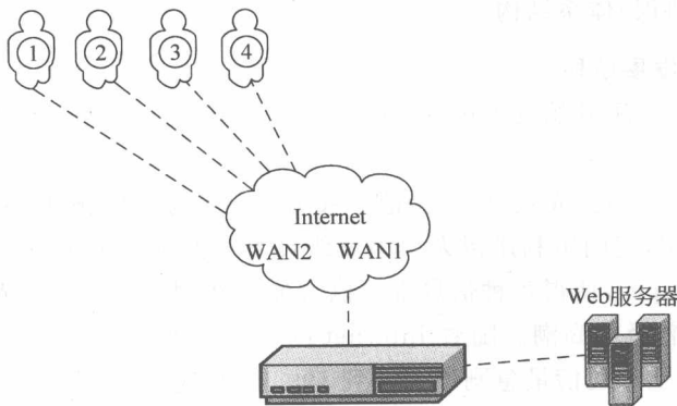
图 1-5 负载均衡原理图
