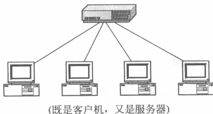
图 1-9 对等网
