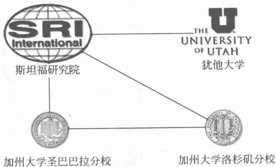
图 1-3 ARPANET 网
