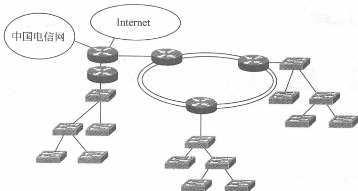
图 1-7 城域网
