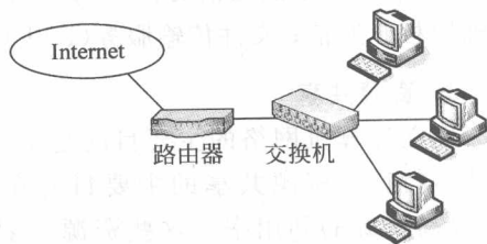
图 1-6 局域网
