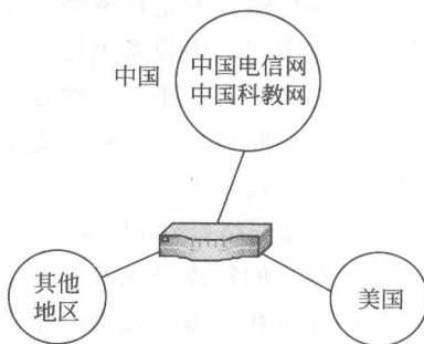
图 1-8 广域网
