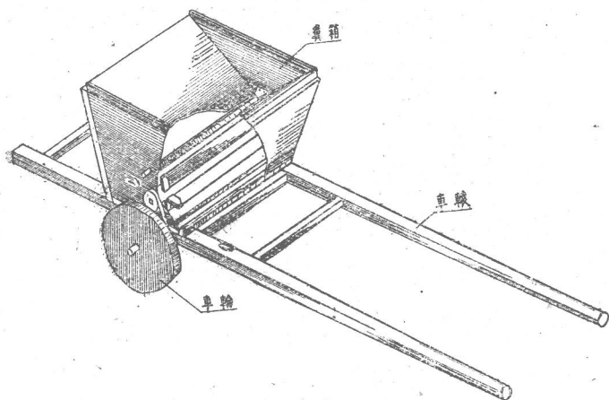
拉糞撒糞車
