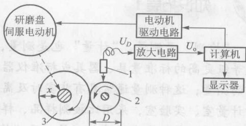
图 1-2 工业检测控制系统
