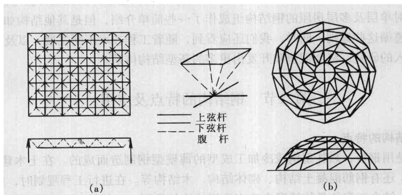
图 1-3 空间屋盖结构
