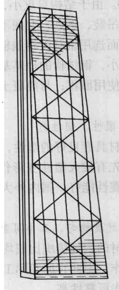
图 1-6 钢支撑筒结构
