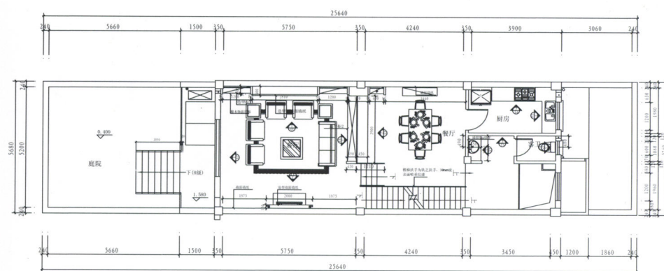
一层平面图
