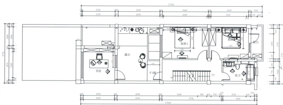
二层平面图
