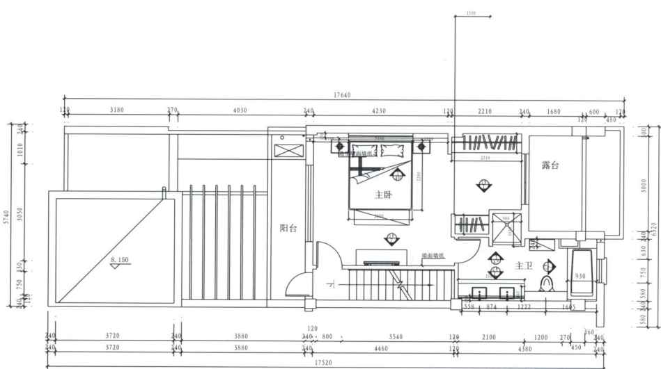
三层平面图
