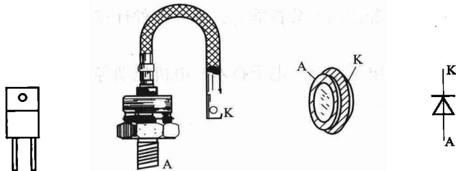
图 1-1 功率二极管的外形及电气符号
