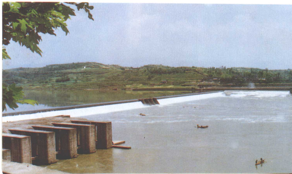
◀ 南阳滩水电站闸坝工程
