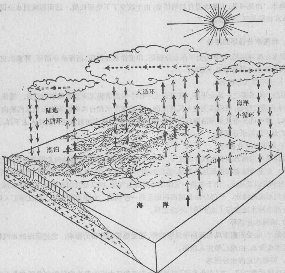
图 1-1 水分循环示意图
