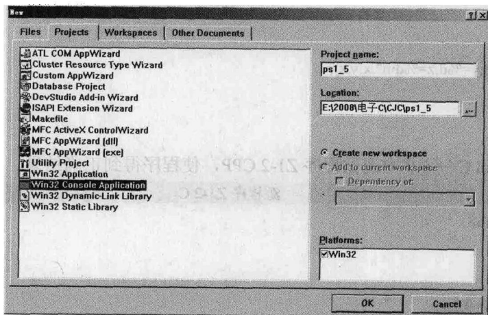
图 1.2 “New”对话框
