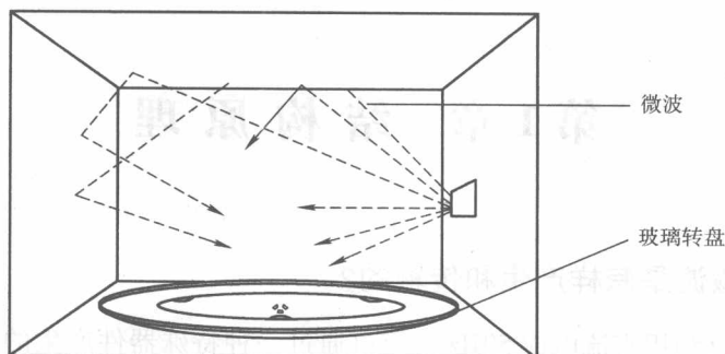
图 1-2 微波加热示意图
