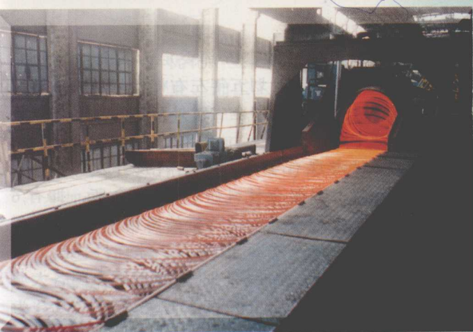
酒钢高速线材生产线
