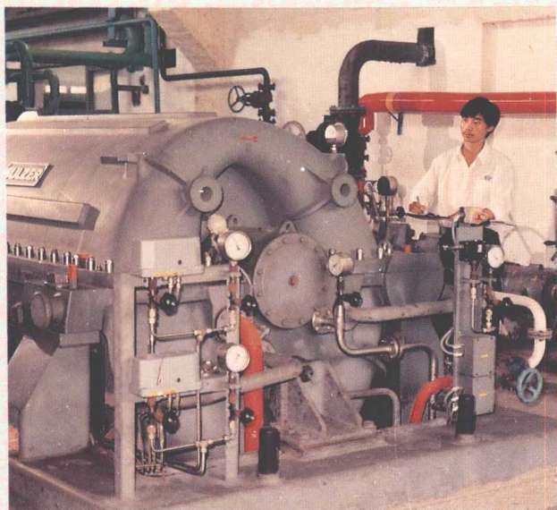
张家坝制盐化工厂热泵制盐
