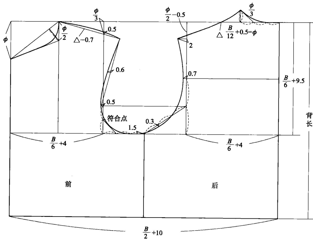
图 1-9 第三代男装基本纸样
