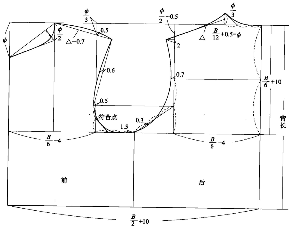
图 1-10 第四代男装基本纸样
