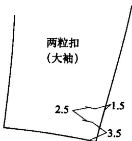
图 1-12 suit 四开身纸样及袖子
