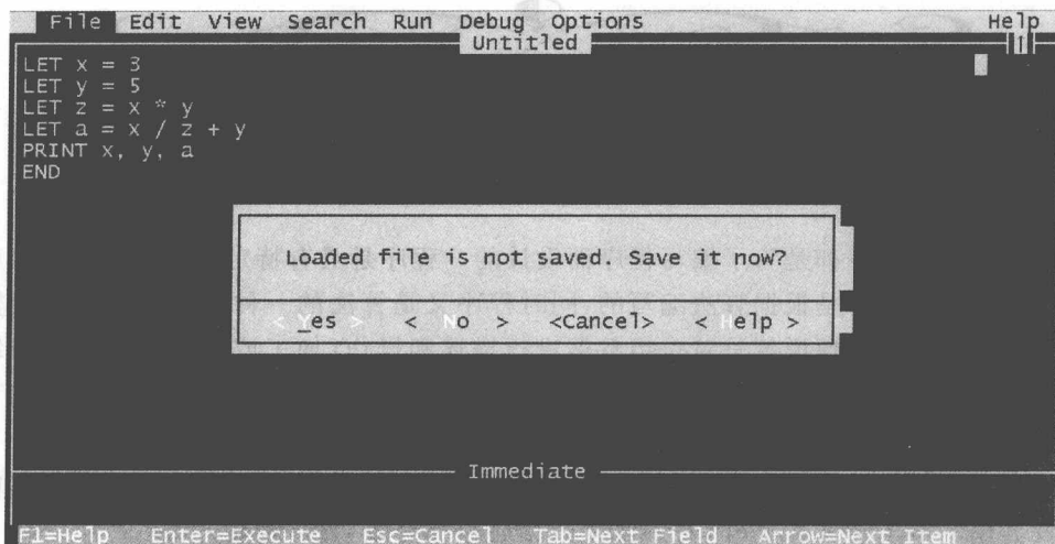
图 1.6 退出 QBASIC
