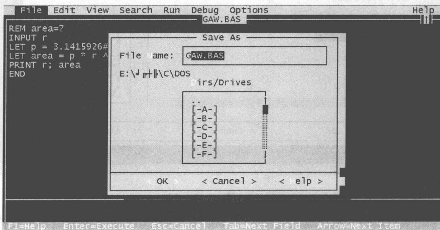
图 1.5 保存文件
