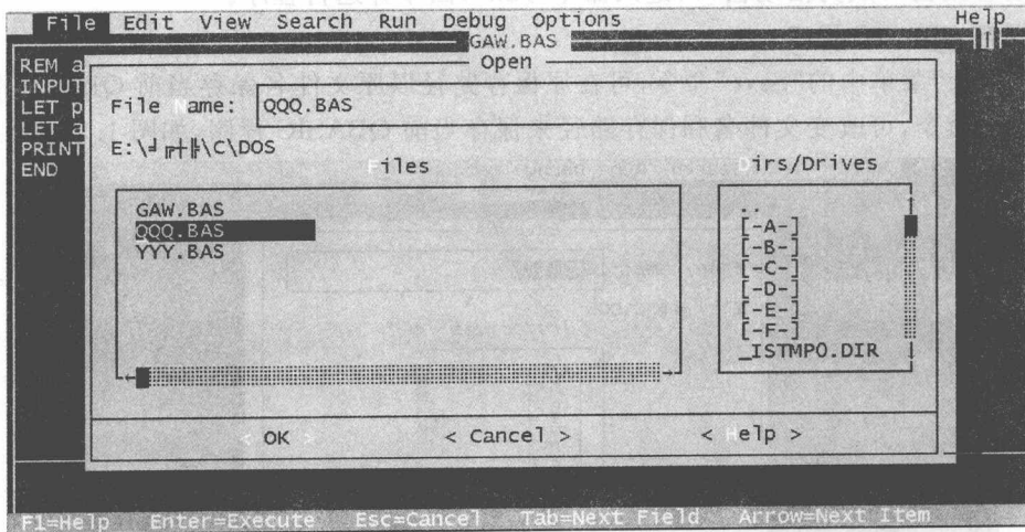
图 1.3 “Open”对话框
