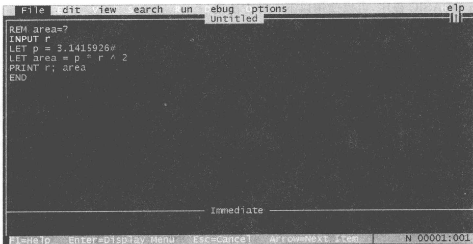
图 1.2 输入程序
