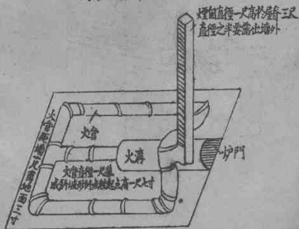
烤房內藏管佈置圖
