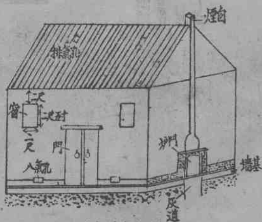
烤房內藏管佈置圖
