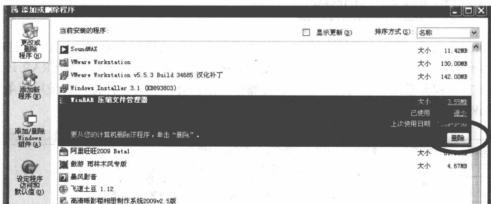
图 1-6-4 程序列表
