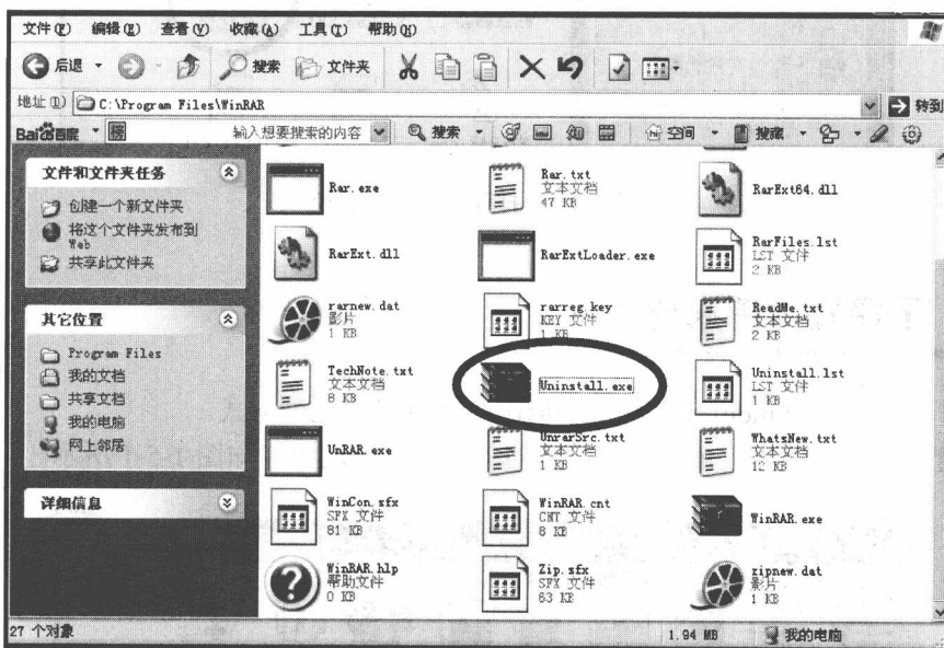
图 1-6-1 卸载程序
