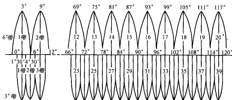
图 1-6 6°带和3°带投影
