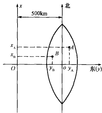
图 1-7 高斯平面直角坐标
