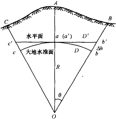
图 1-11 水平面代替水准面的影响
