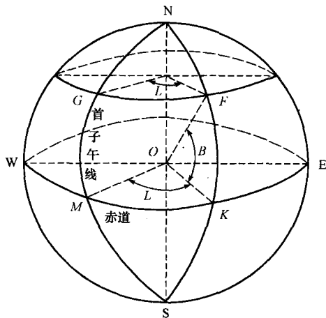
图 1-2 大地坐标系
