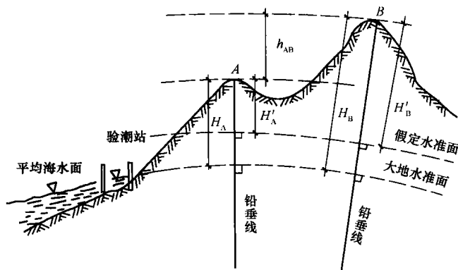
图 1-10 高程和高差
