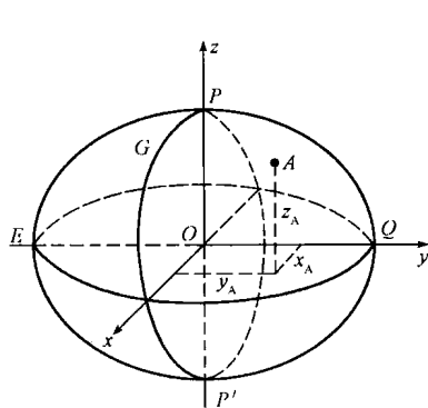
图 1-3 地心坐标系
