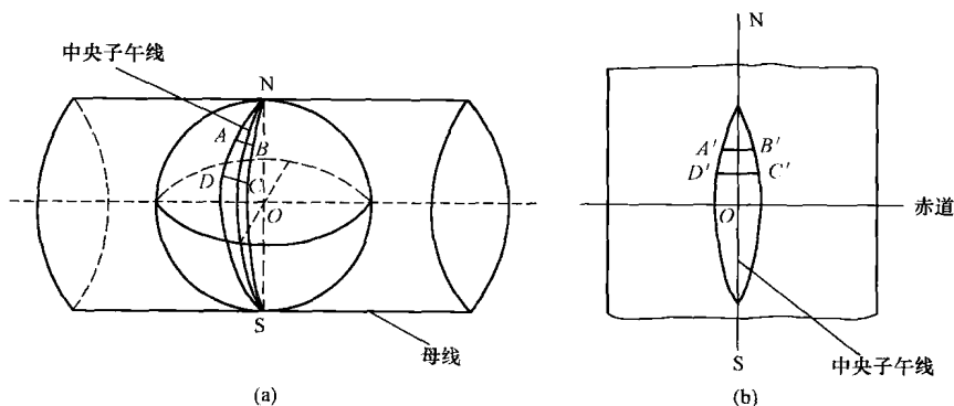
图 1-5 高斯投影
