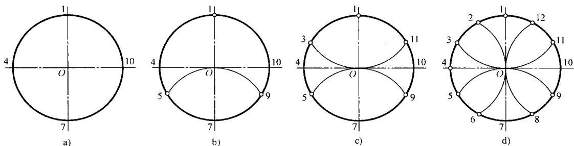
图 1-12 圆的三、六、十二等分法
