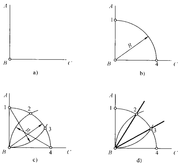
图 1-8 直角的三等分法
