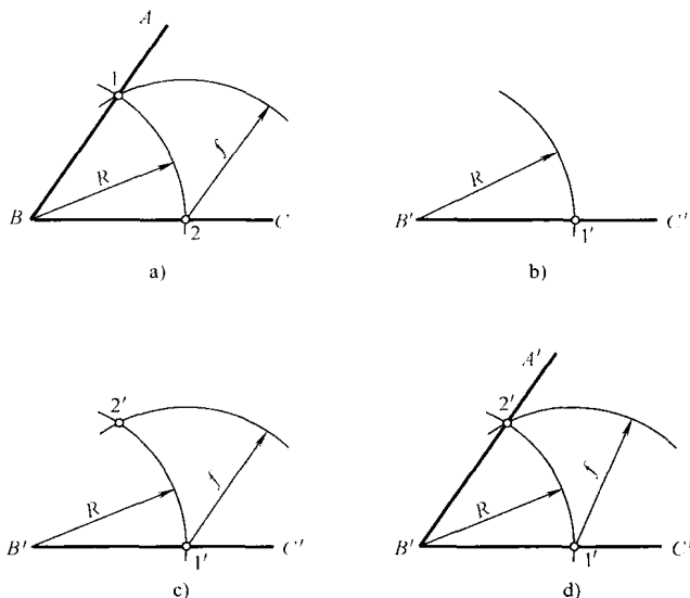
图 1-10 作一角等于已知角
