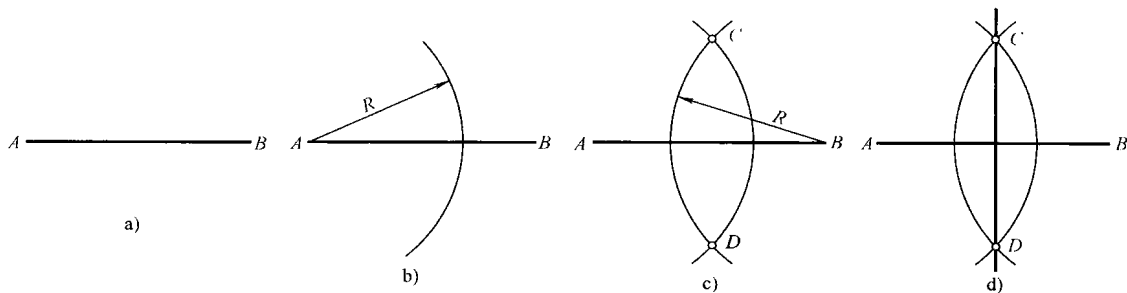
图 1-1 垂直平分线的画法 (a、b、c、d 为作图顺序)
