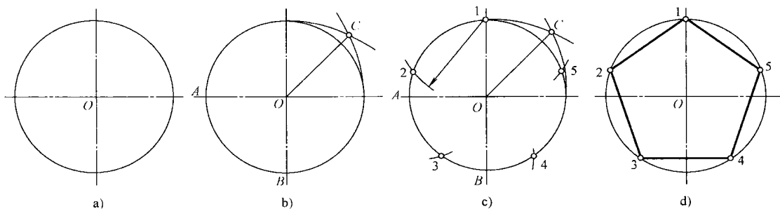
图 1-13 圆的五等分法并作内接正五边形 (方法一)
