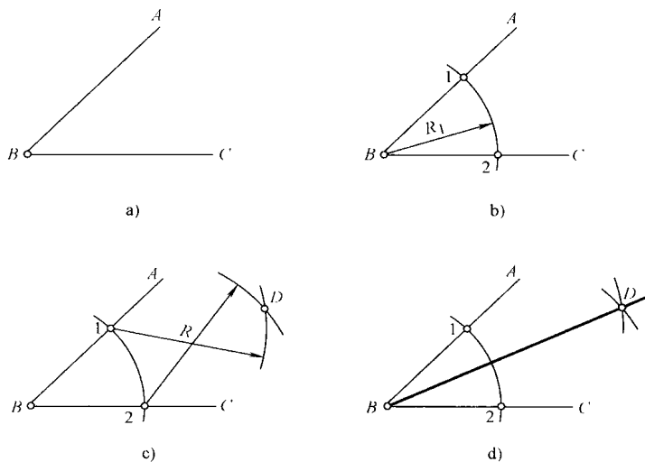
图1-6 任意角的二等分法 (a、b、c、d为作图顺序)
