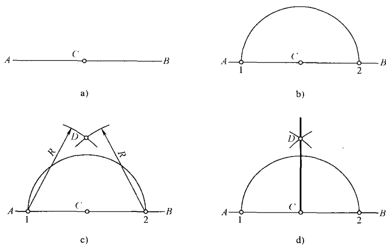
图 1-2 由直线上的定点作该线的垂线 (a、b、c、d 为作图顺序)
