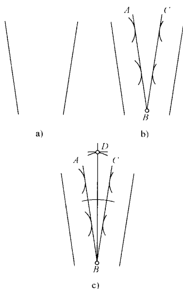
图 1-7 无顶角的二等分法
