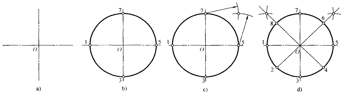
图 1-11 圆的四、八等分法
