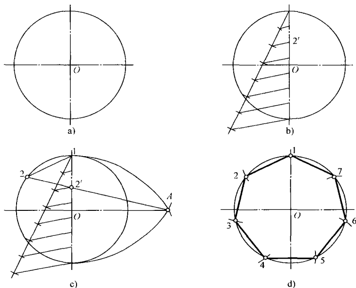
图 1-15 圆的任意等分法
