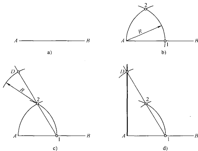
图 1-3 过线端点作垂线法 (a、b、c、d 为作图顺序)
