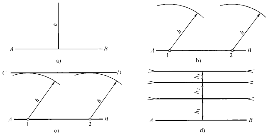
图 1-4 平行线画法 (a、b、c、d 为作图顺序)
