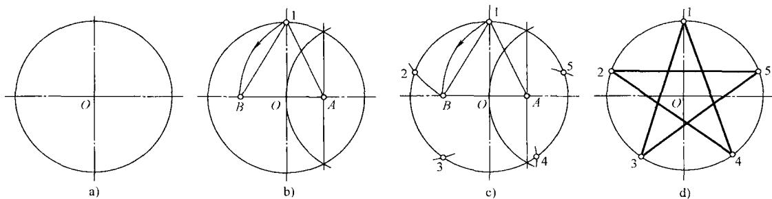
图 1-14 圆的五等分法并作圆内五角星（方法二）
