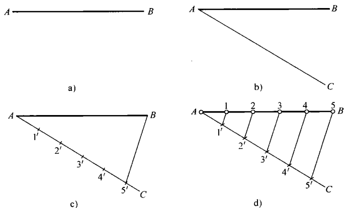
图 1-5 线段五等分法 (a、b、c、d 为作图顺序)
