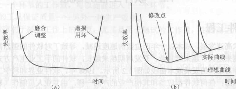
图 1.1 失效率曲线
