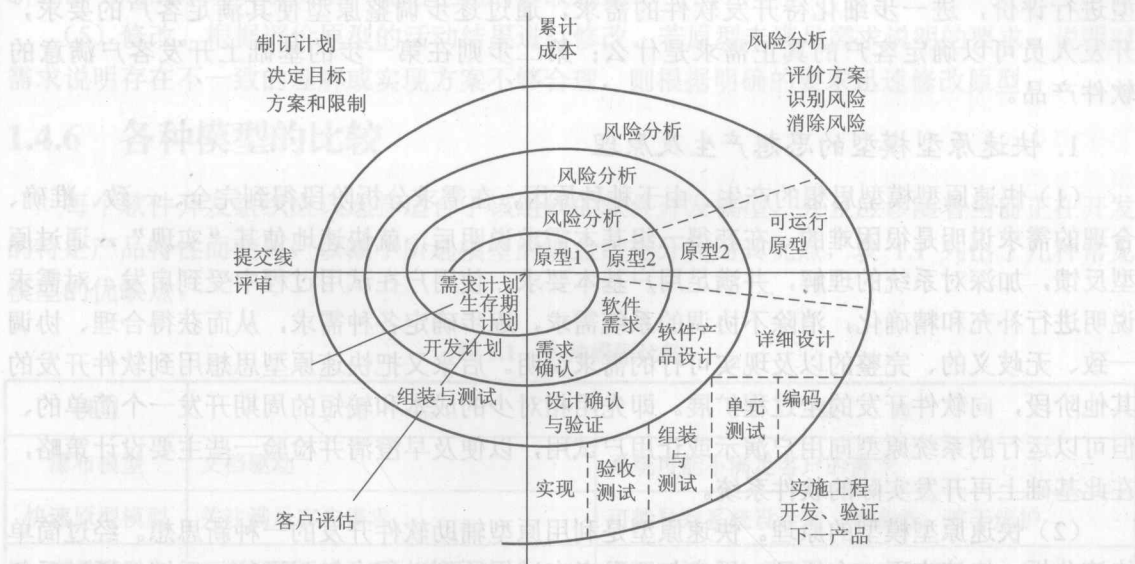
图 1.6 螺旋模型
