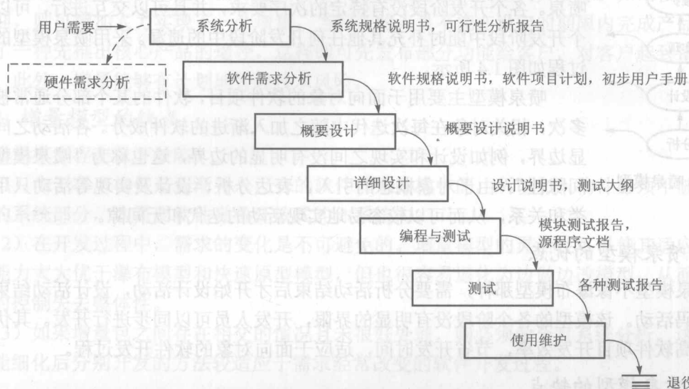
图 1.3 瀑布模型
