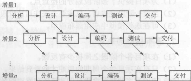
图 1.5 增量模型
