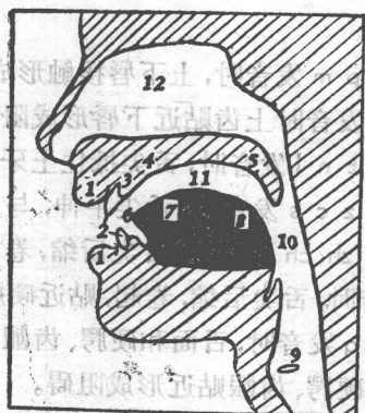
语音器官图
