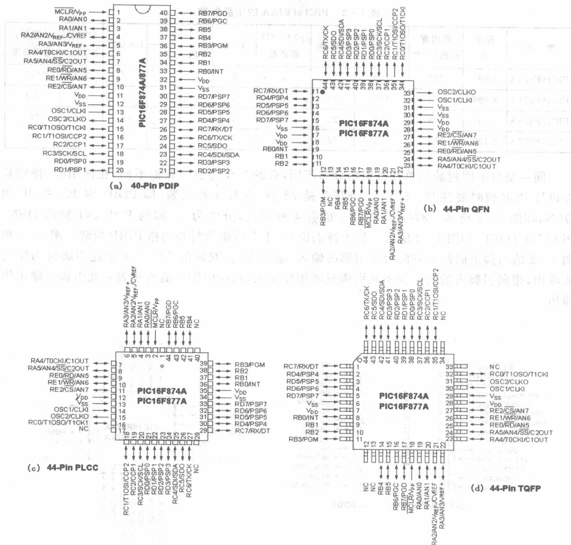
图 1-2 874A 与 877A 的不同封装引脚图
