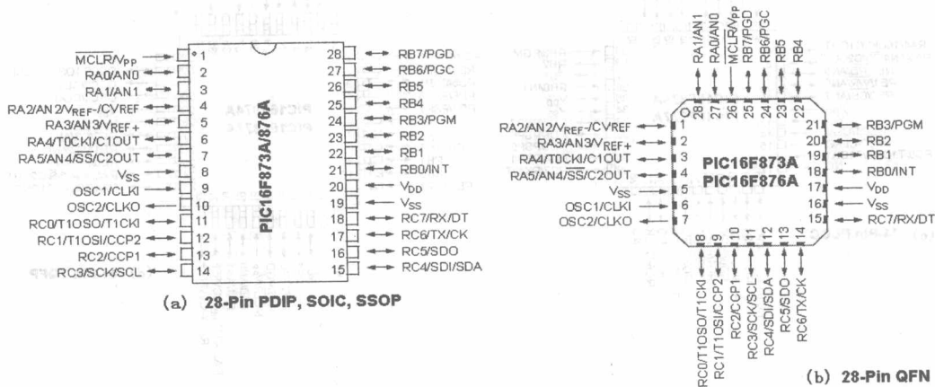
图 1-1 873A 与 876A 的不同封装引脚图
