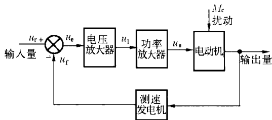
图 1-7 直流电动机转速闭环控制系统方块图
