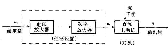
图 1-5 直流电动机转速开环控制系统方块图
