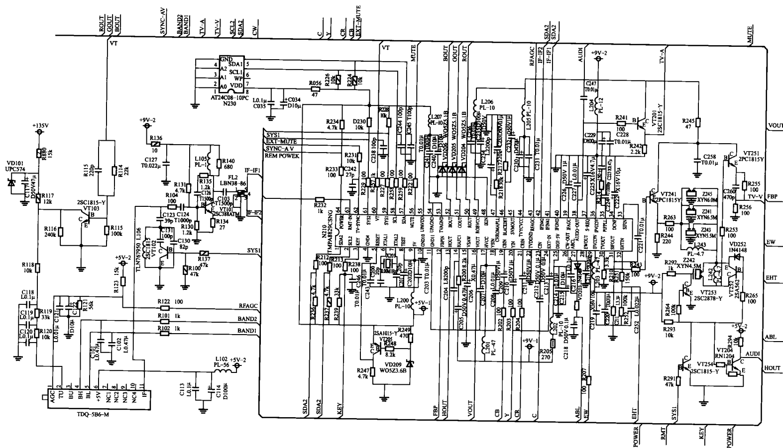
图 1-8 长虹 PF2991E 电视机超级芯片电路
