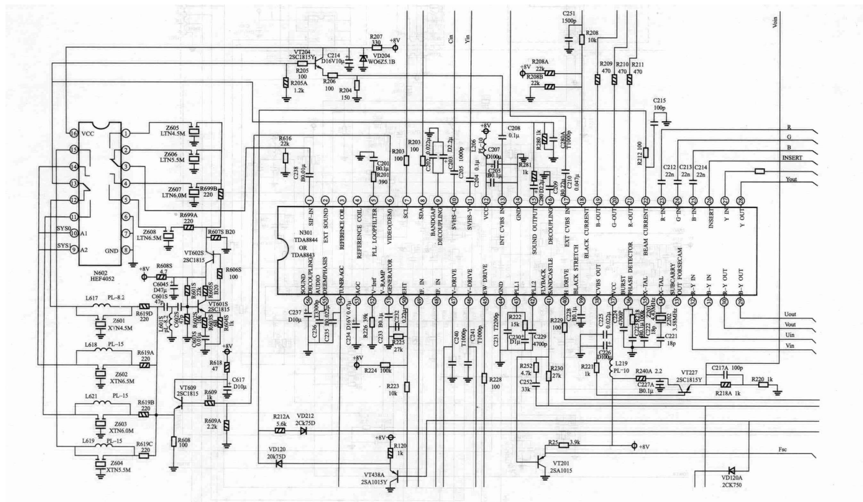
图 1-1 长虹 CH-10DR 机芯 (H29D80) 电视机单片小信号处理电路
