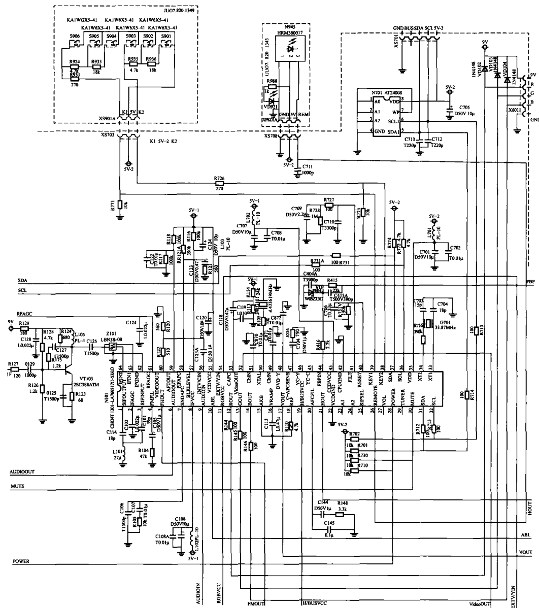
图 1-2 长虹 CH-13A 机芯 (SF2129K) 电视机超级芯片电路
