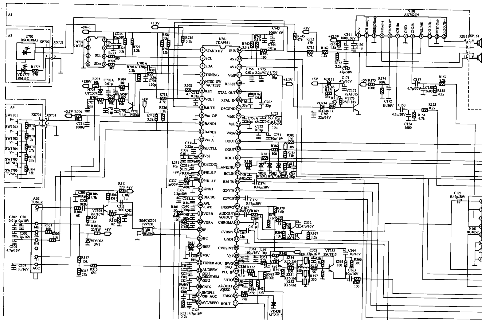
图 1-6 长虹 PE3495AST 电视机超级芯片电路
