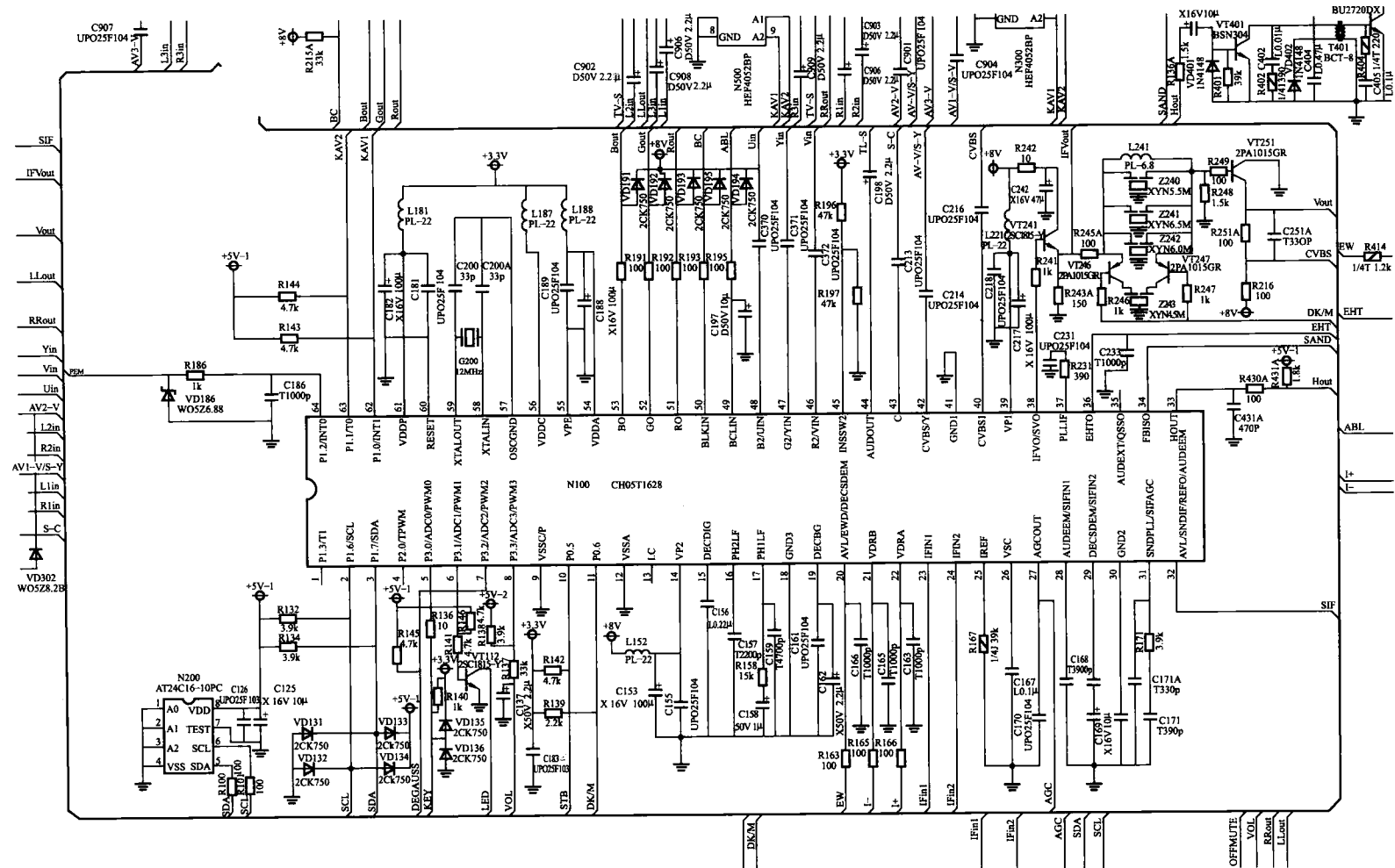
图 1-7 长虹 PF29118 电视机超级芯片电路
