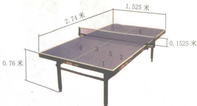
图 1-1-1 球台规格
