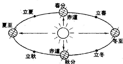
八个节气图
