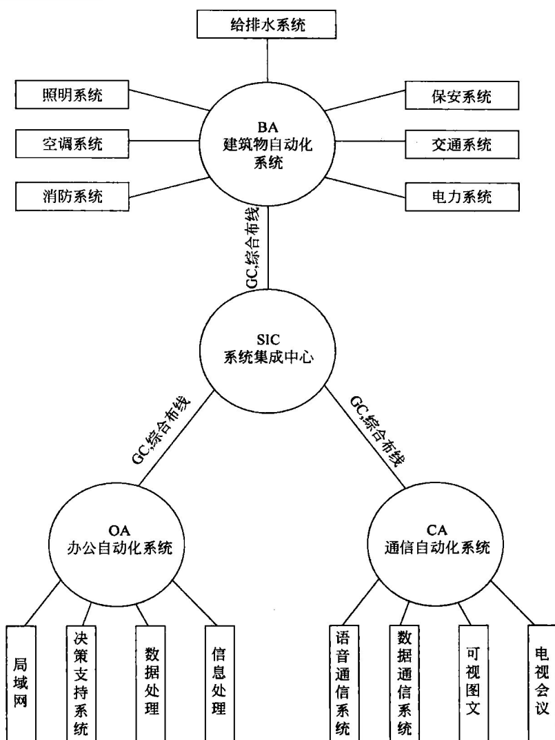
图 1-1 智能大厦的组成结构
