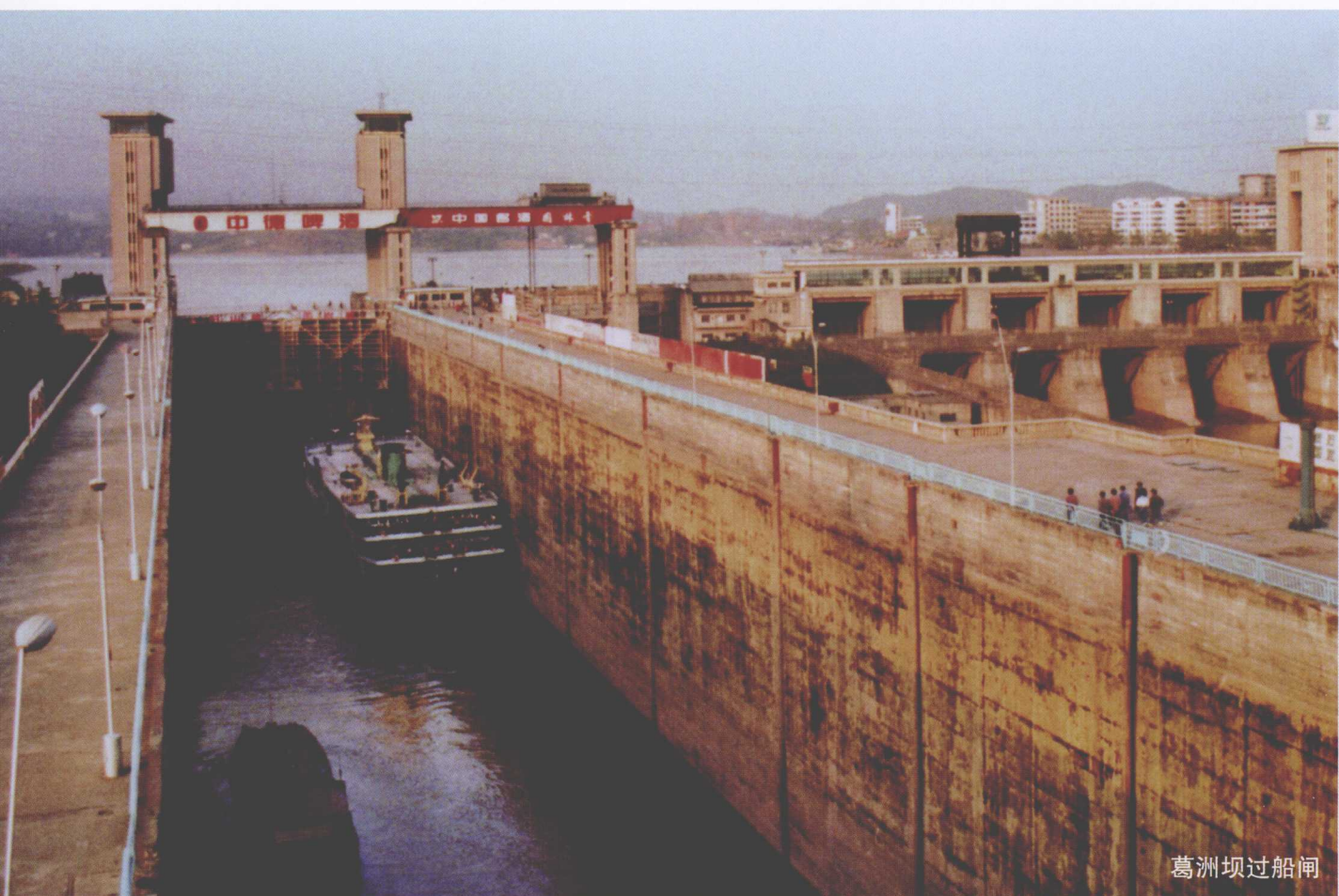
葛洲坝枢纽航运工程是“两线三闸”。自1981年6月通航以来，作为配合三峡工程建造的调节航运梯级工程，极大地改善了长江三峡区域120公里水域的通航条件，大量货船从此安全畅通地出入川江。
