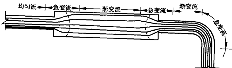
图 10-3 均匀流和不均匀流
