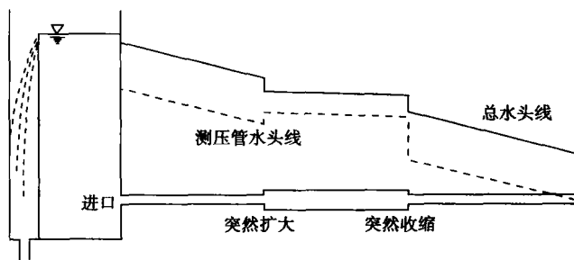
图 10-4 总水头线和测压管水头线
