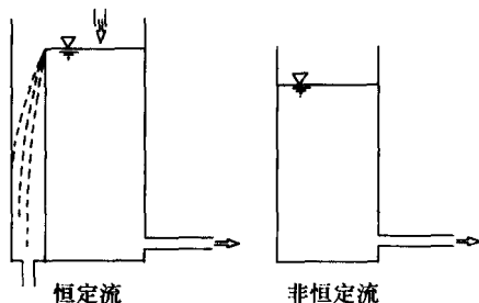
图 10-1 恒定流与非恒定流
