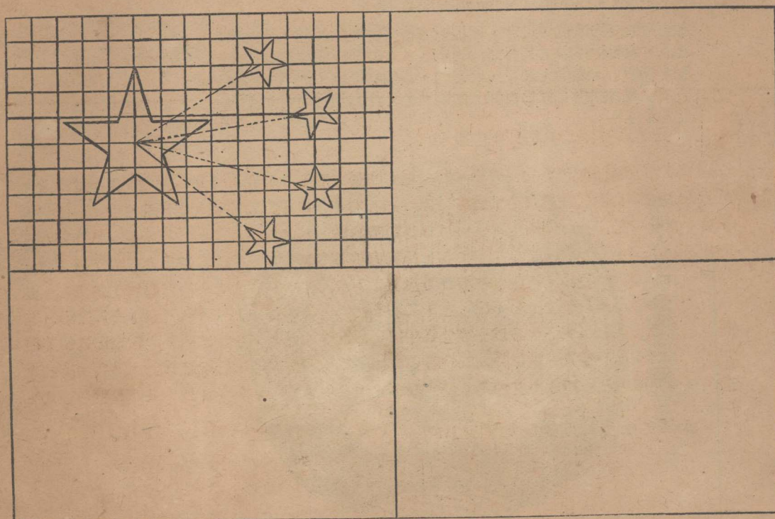
中華人民共和國國旗製作圖
