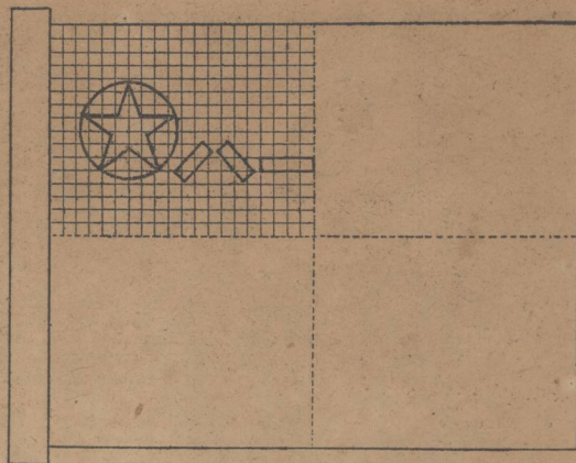
中國人民解放軍軍旗製作圖
