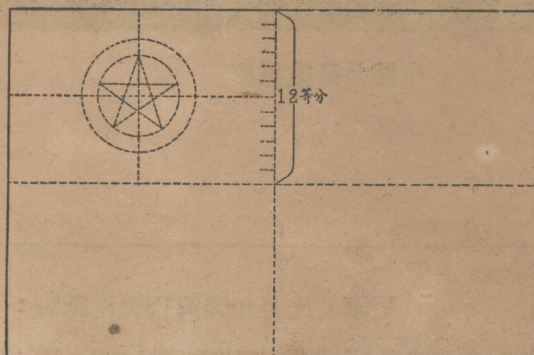
中國新民主主義青年團團旗製作圖
