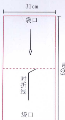
背囊结构图
