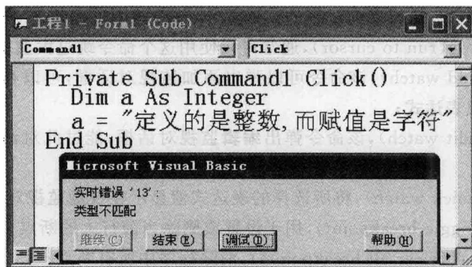
图 1.4 运行错误
