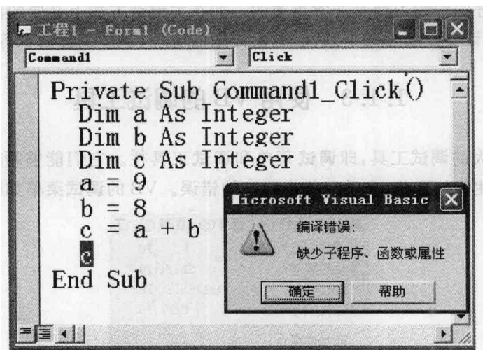
图 1.3 编译错误
