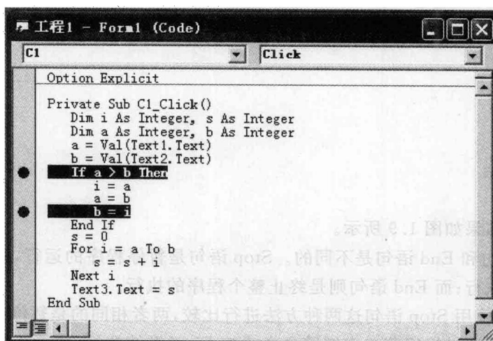
图 1.7 设置断点
