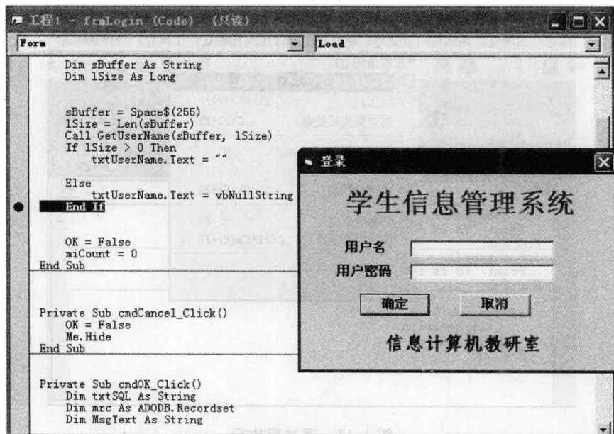
图 1.10 逐语句执行
