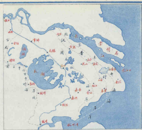
太湖地区成陆年代
