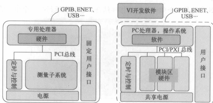
图1-3 传统仪器（左图）与虚拟仪器（右图）的比较
