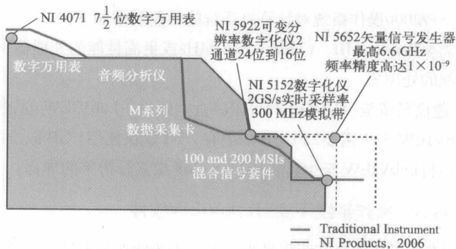
图1-6 虚拟仪器与传统仪器硬件性能的比较
