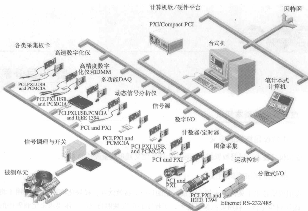
图1-2 虚拟仪器系统的组成
