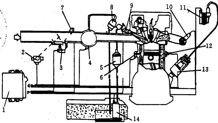
图 2-2 电喷式发动机系统的原理图
