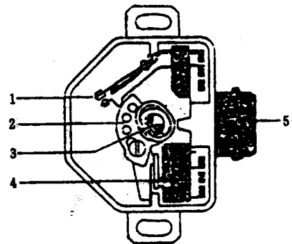
图 2-5 节气门位置传感器
