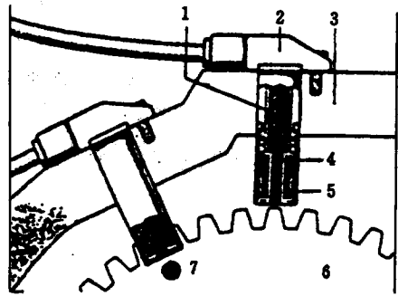
图 2-4 发动机转速传感器和曲轴位置传感器 1-永久磁铁;2-固定外壳;3-发动机机体;4-铁芯; 5-电磁感应线圈;6-飞轮;7-基准位
