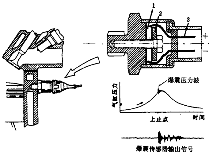
图 2-9 爆震传感器
