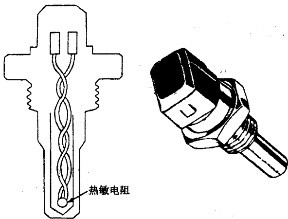
图 2-6 发动机冷却液温度传感器
