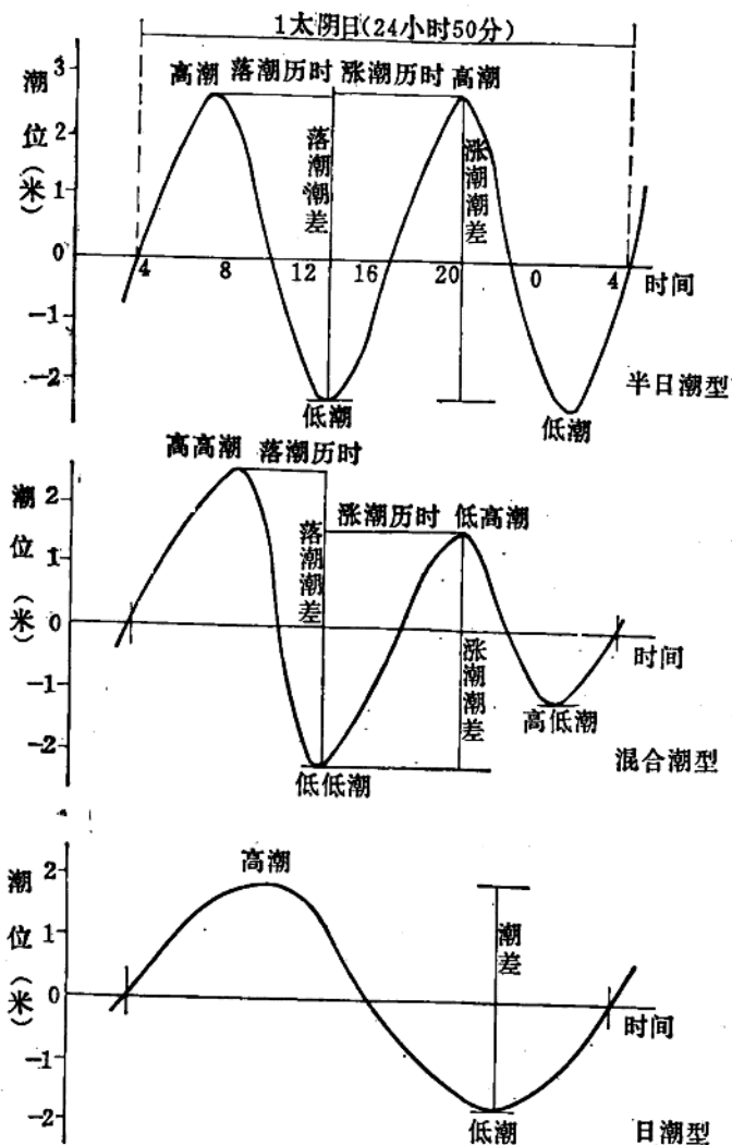
图 1-3 潮汐涨落三种类型工程特征值图
