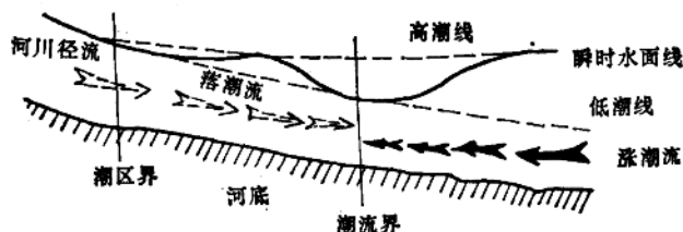
图 1-2 河口潮汐的“潮流界”和“潮区界”
