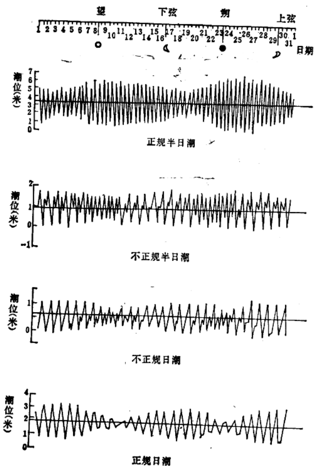
图 1-1 潮汐类型
