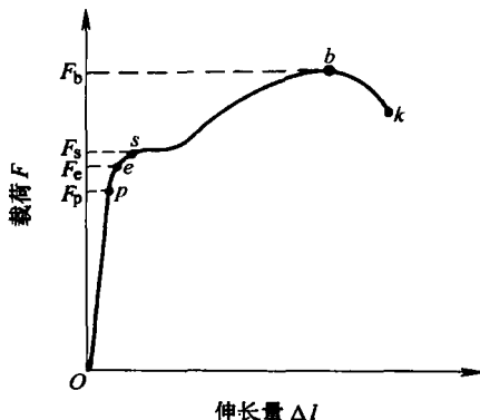
图 1-2 低碳钢的拉伸曲线
