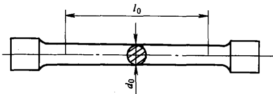
图 1-1 标准拉伸试样
