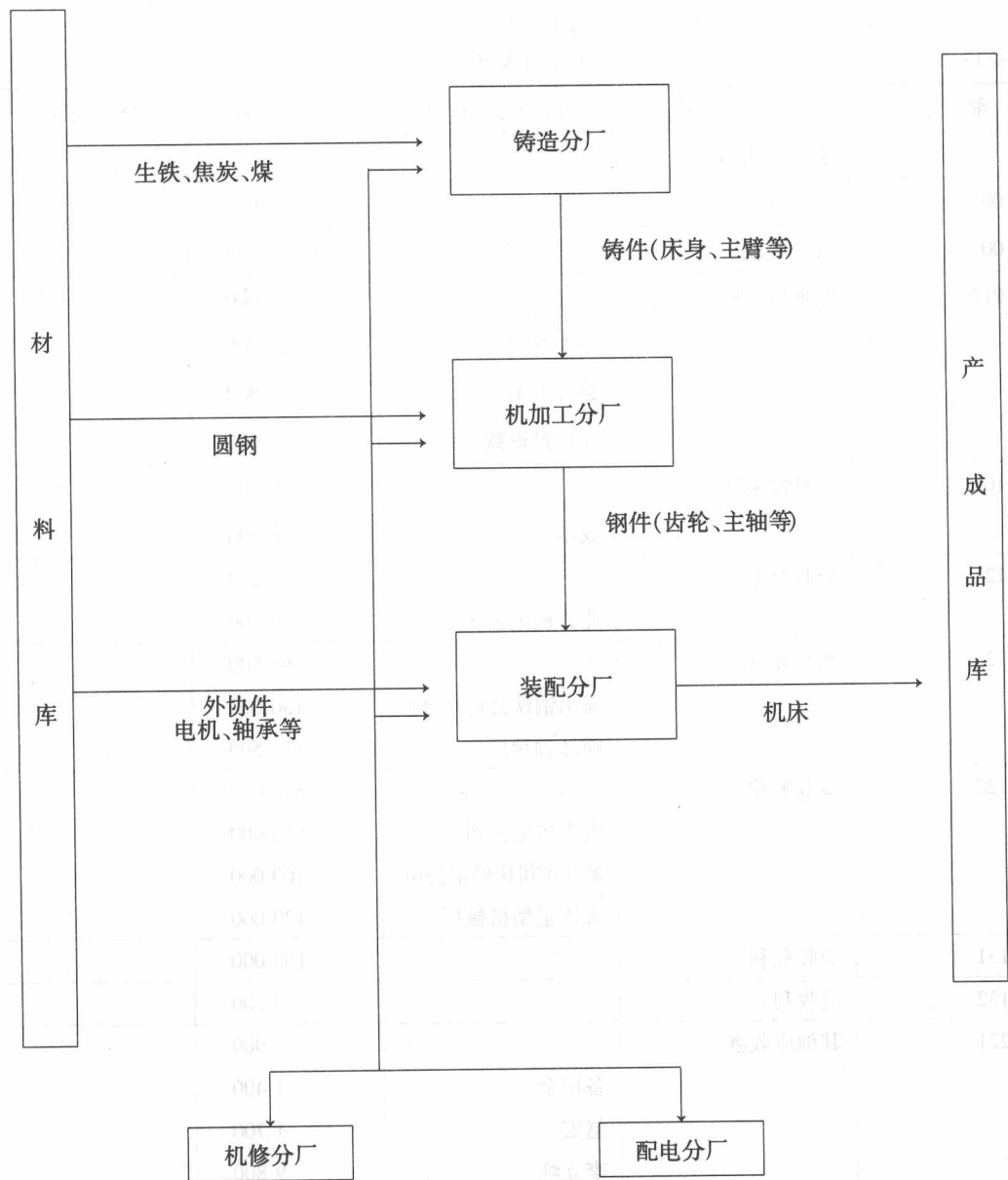
图 1—3 生产工艺流程图
